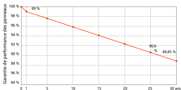
Performance linéaire garantie 30 ans
