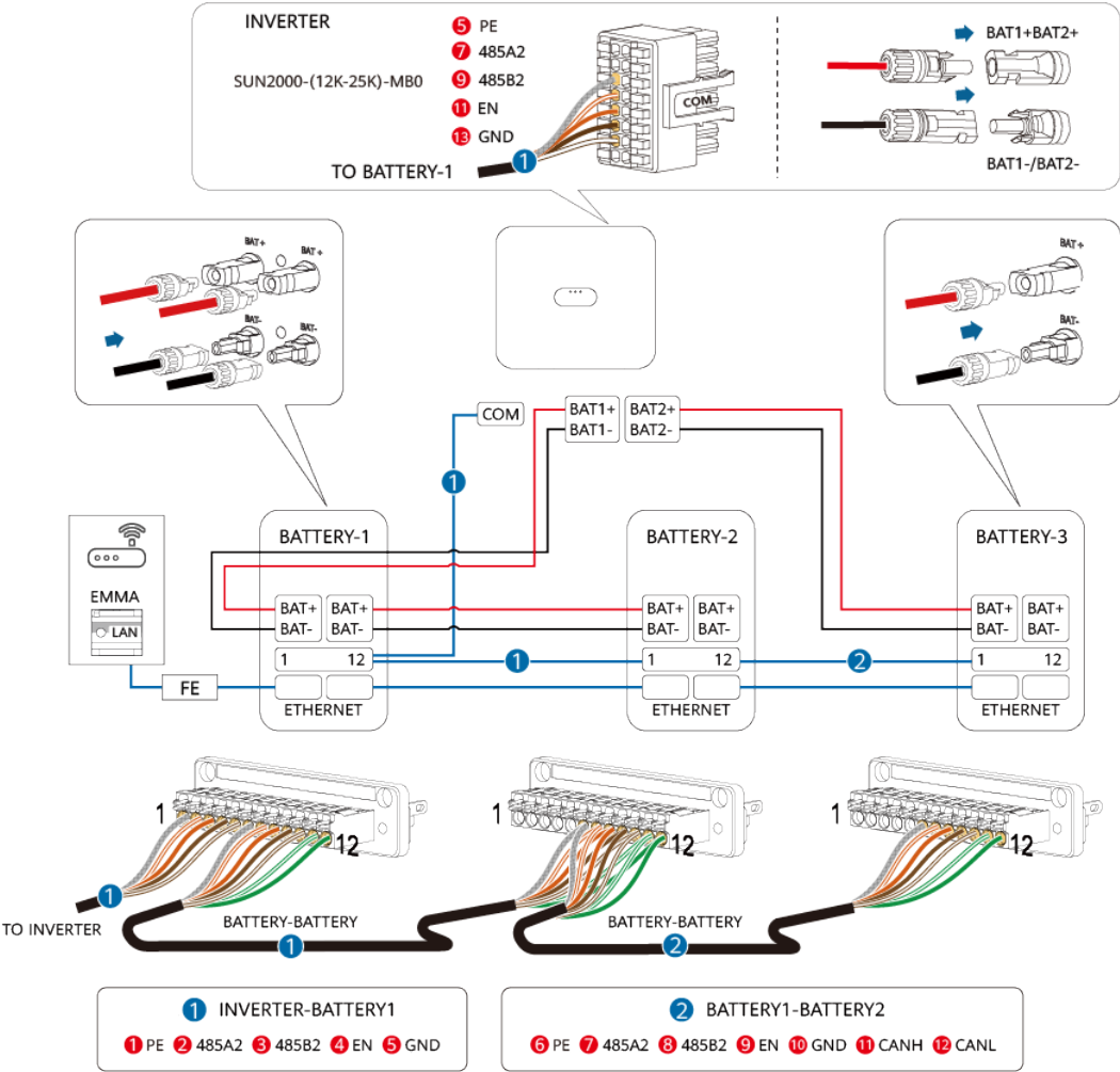
Figure 5-10 Onduleur connecté à trois ESS
