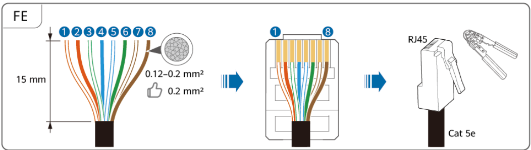
Figure 5-6 Préparation du câble réseau
