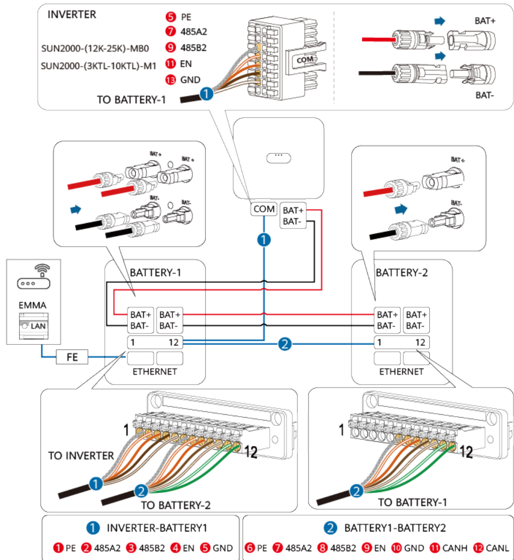
Figure 5-9 Onduleur connecté à deux ESS
