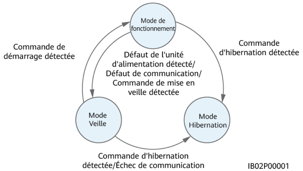
Figure 2-17 Changement de mode de fonctionnement
